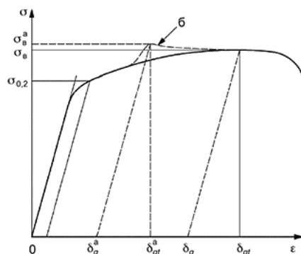
а - недопустимые значения, полученные в результате внезапного увеличения скорости деформации; б - поведение диаграммы "напряжение - деформация" при внезапном увеличении скорости деформации
